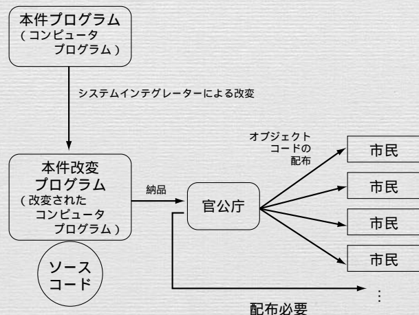
図2 市民利用の場合におけるソースコード配布の必要性
