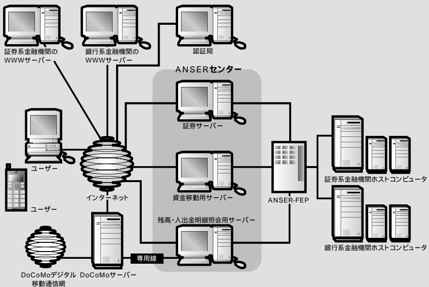
ANSER-WEBのシステム構成図
