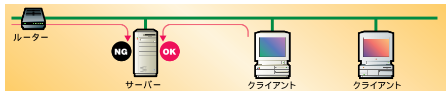
図 tcp-wrapperの働き
