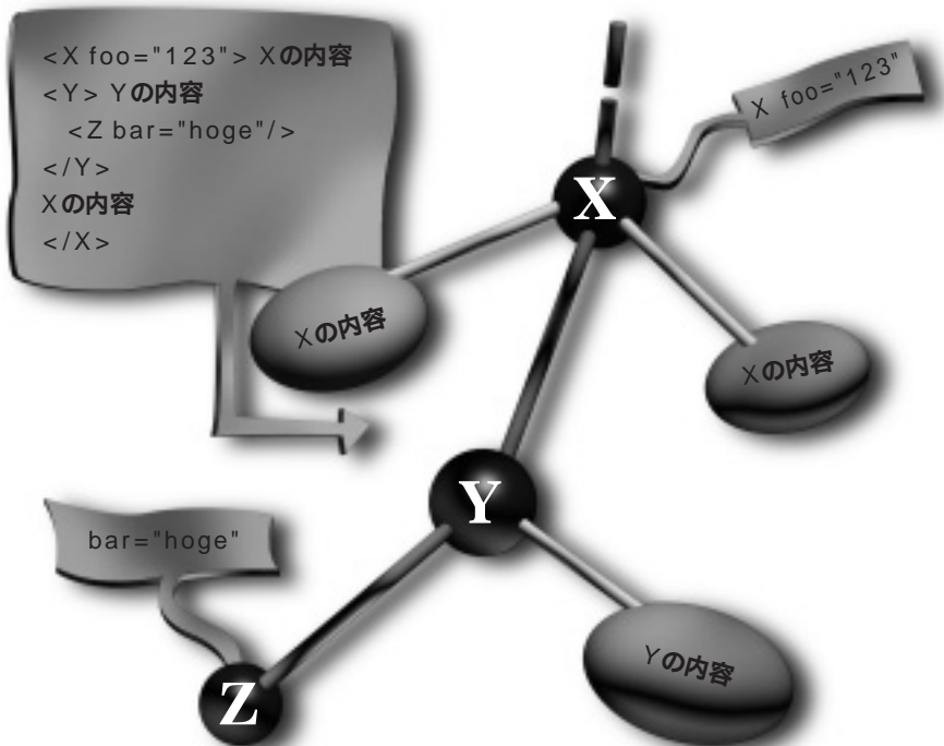
図4 知らないタグでもツリーを構成できる。
